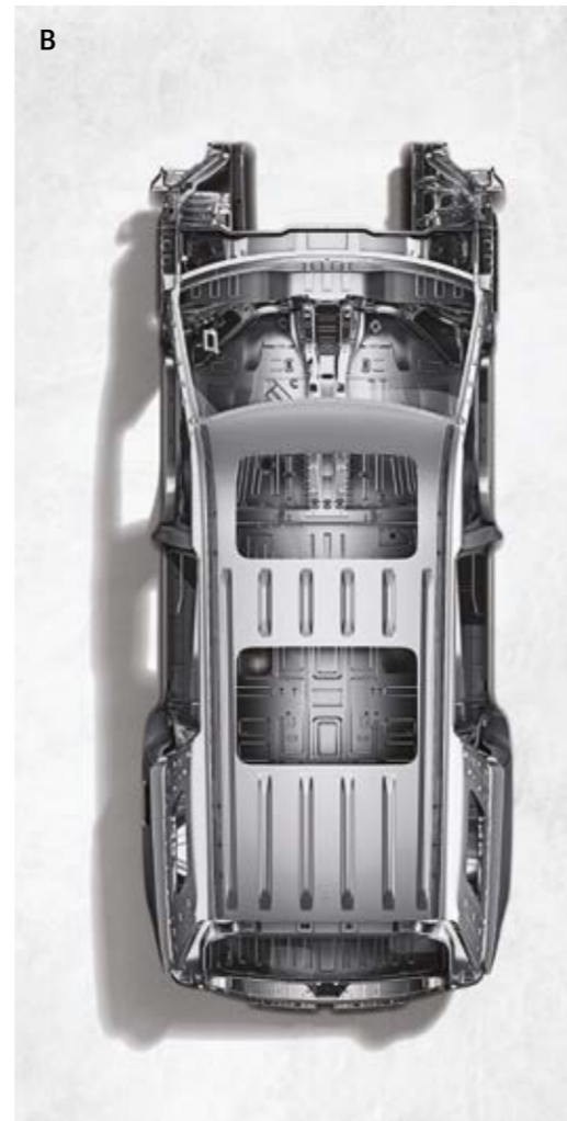
B. חומרים חכמים יותר במרכב והשלדה יישומים חדשים של פלדה חזקה יותר ונוחה יותר לעיבוד באזורים קריטיים, מסייעים למרכב ולשלדה לפזר טוב יותר את כוחות ההתנגשות כדי לשפר את ההגנה על הנוסעים. קשיחות פיתול גבוהה יותר מספקת התנהגות כביש בעלת רמת היענות מרשימה ונסיעה חלקה להפליא.
