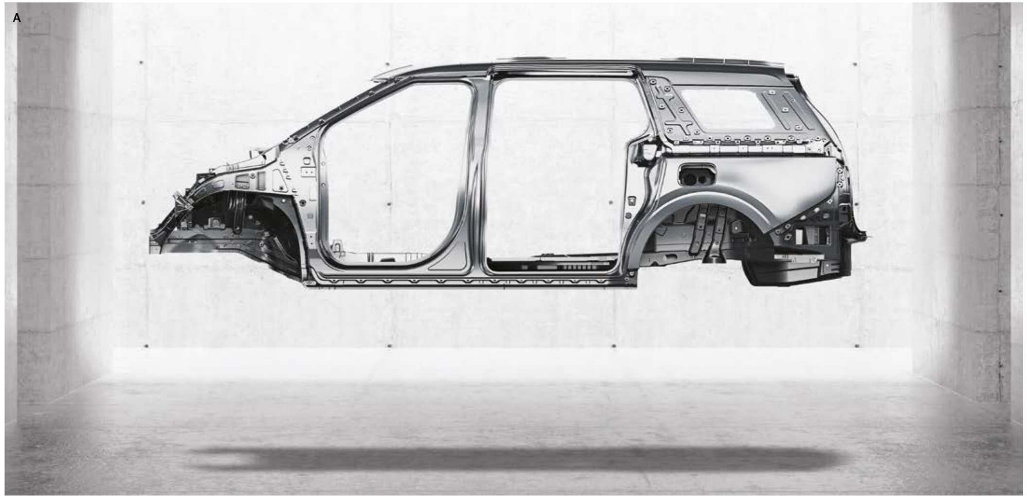
A. פלטפורמה מהדור השלישי בפלטפורמה מהדור השלישי נעשה ארגון מחדש של מערכת ההיגוי, השלדה, חטיבת ההינע ורצפת תא הנוסעים, לקבלת תא נוסעים מרווח יותר וביצועי אווירודינמיים, התנהגות כביש, יציבות ובטיחות בהתנגשות טובים יותר. הקרניבל נהנה מההתקדמות שנעשתה בכל מערך הדגמים של קיה.
